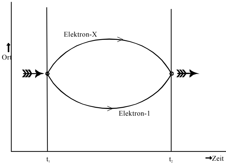
Bild 10: Zeitschleife eines Elektrons
