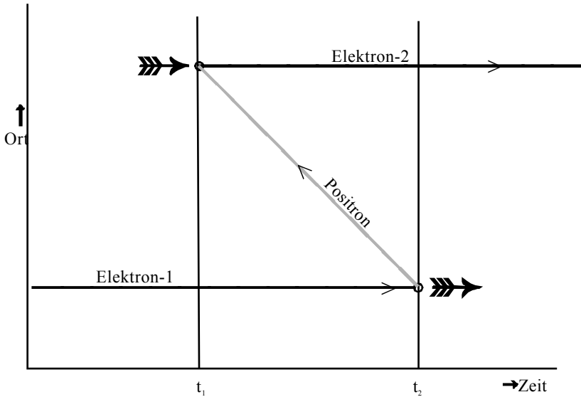
Bild 11: Zeitreise eines Elektrons
