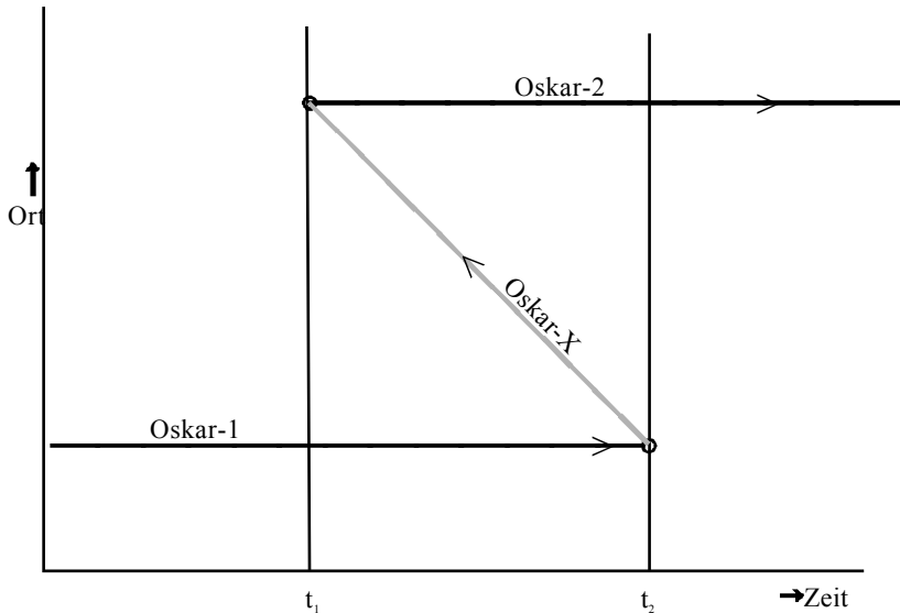
Bild 2: Weltlinie einer Reise in die Vergangenheit . Oskar reist zur Zeit t_2 in die Vergangenheit, kommt zur Zeit t_1 an einer anderen Stelle seines Zimmers an und lebt als Doppelgänger ("Oskar-2") weiter. Als Zeitreisender ("Oskar-X") hat er eine andere Konsistenz; deswegen die andere Farbe dieses Teils der Weltlinie
