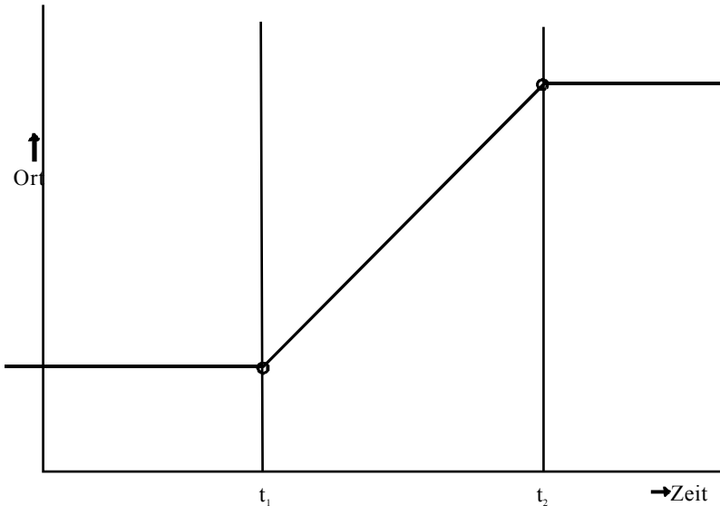
Bild 1: Raum-Zeit-Diagramm. Eingezeichnet ist die Weltlinie eines Objekts, das bis t_1 ruht, dann nach oben rückt und ab t_2 wiederum ruht.
