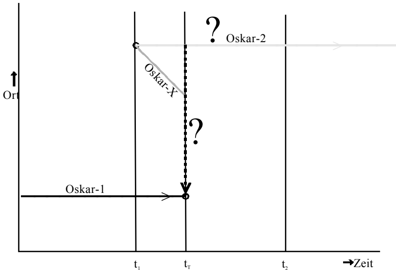
Bild 3: Zeit-Paradoxon. Oskar-2 tötet zur Zeit t_T den Oskar-1 oder hindert ihn an der Zeitreise. Wie aber kann er dann zu Oskar-2 werden?
