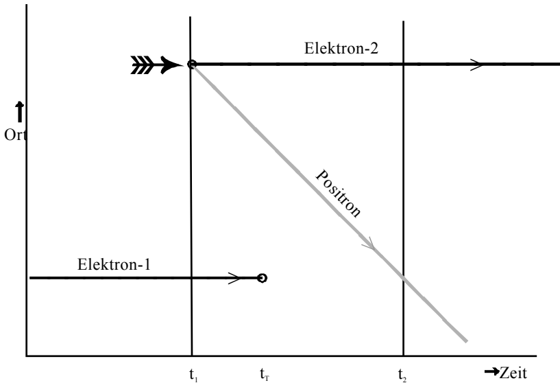
Bild 12: Das Zeitparadoxon mit zwei Elektronen und einem Positron als "Zeitreisendem"
