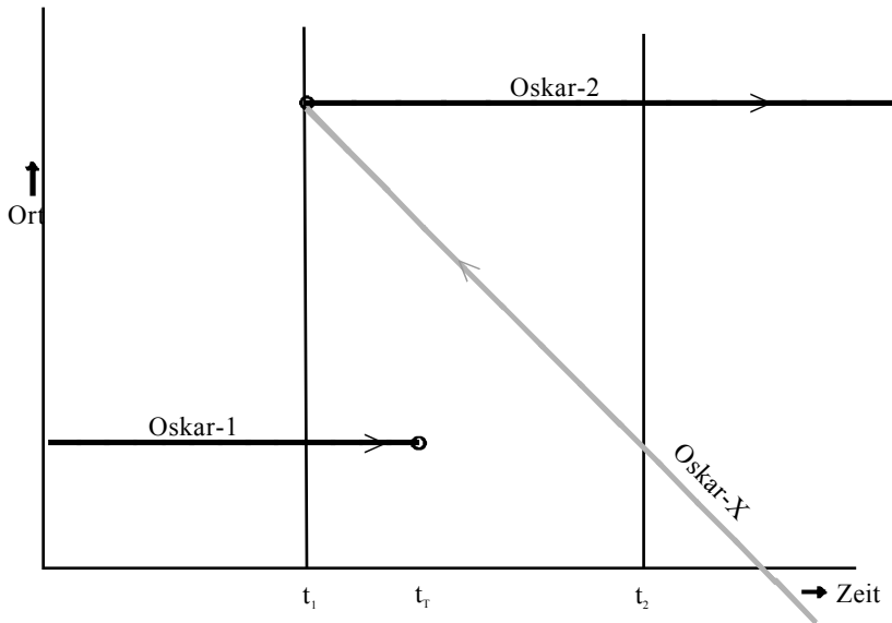
Bild 13: Das Zeitparadoxon gelöst
